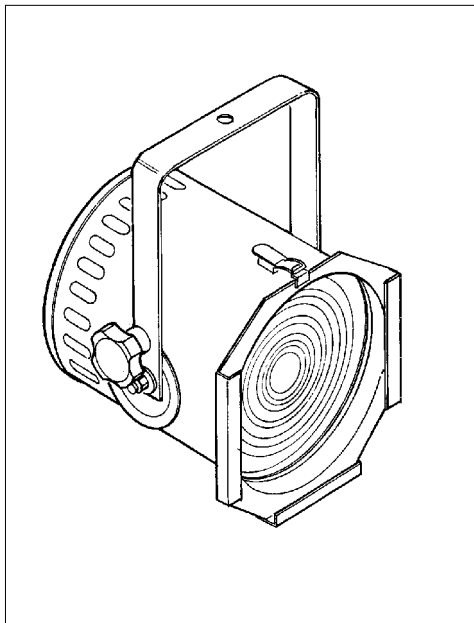
FRESNEL 8"
